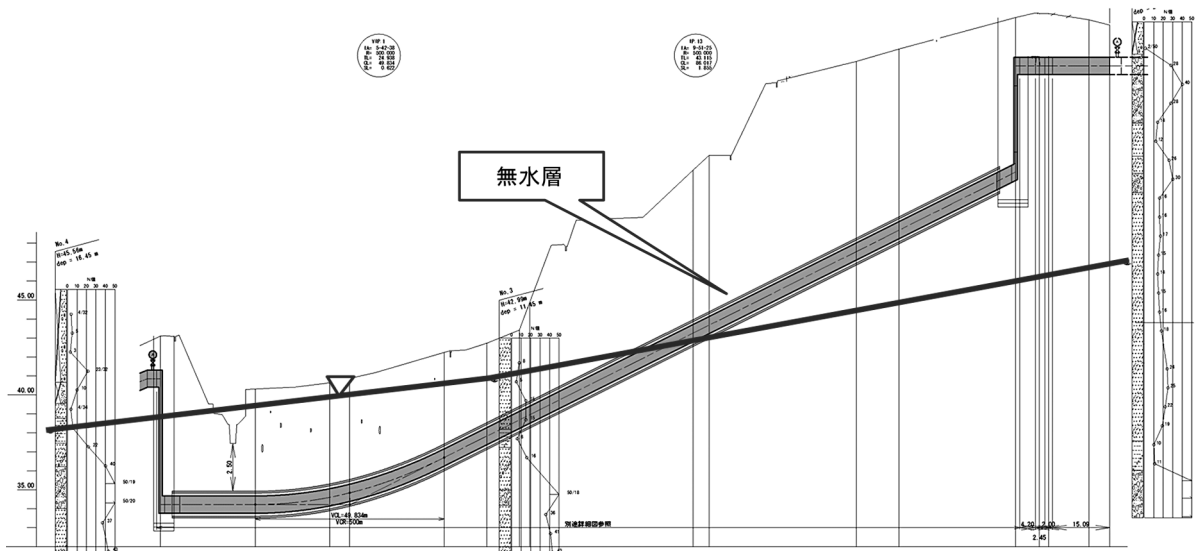
図-2 断面図
